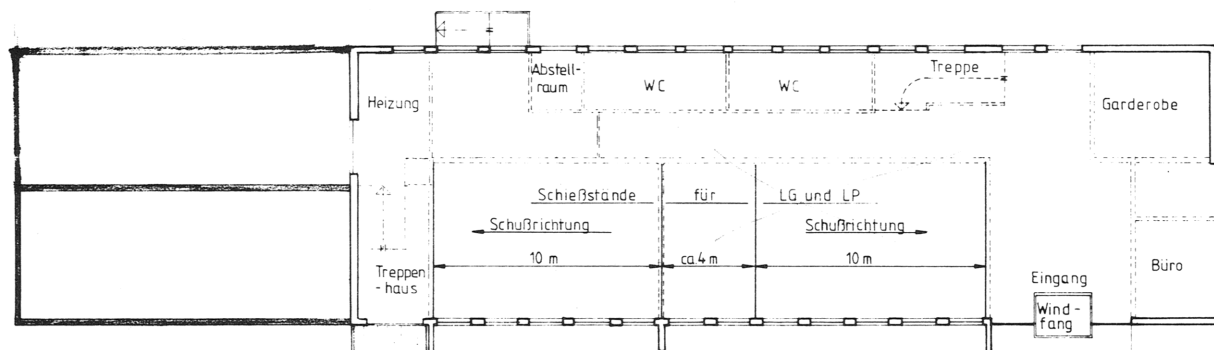
GRUNDRISS ERDGESCHOSS
