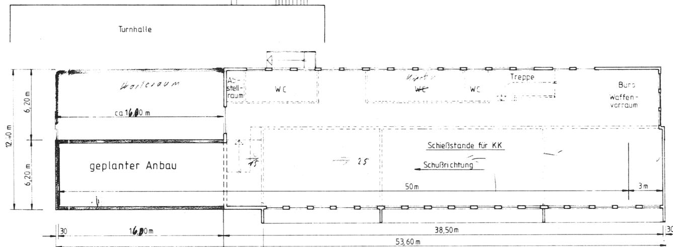
GRUNDRISS OBERGESCHOSS
